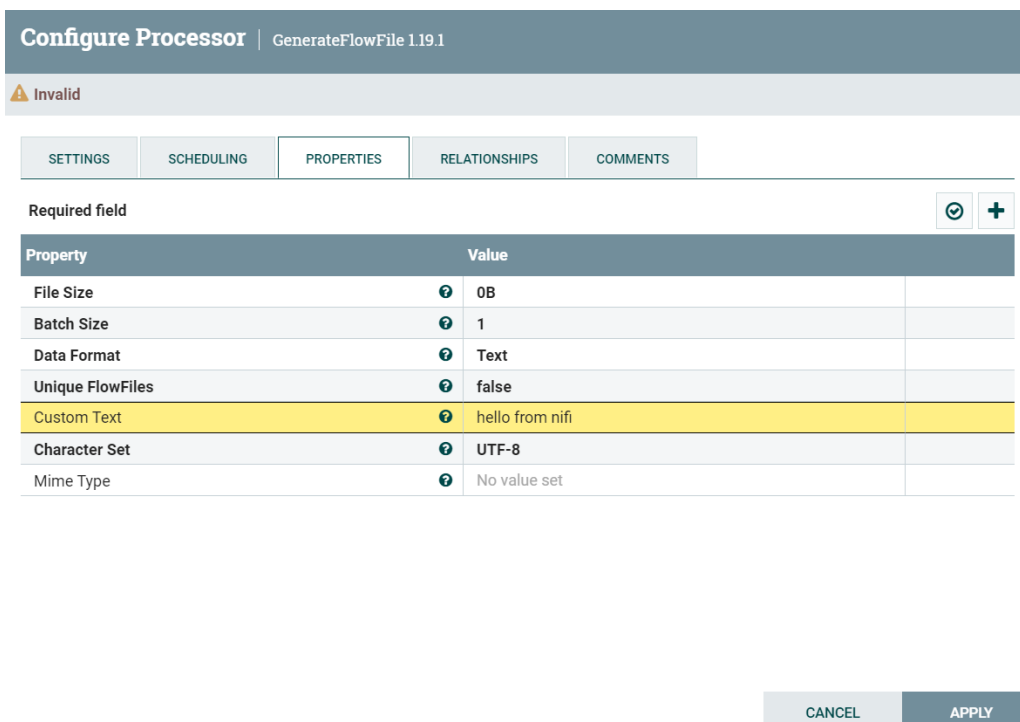
Рисунок 12.14 Properties
