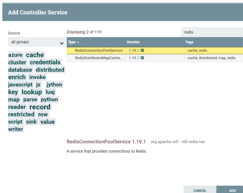
Рисунок 12.2 Redis
