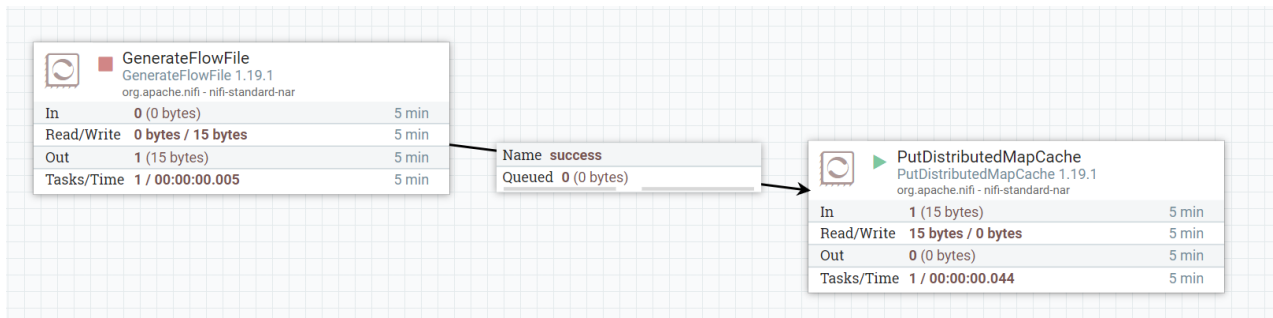
Рисунок 12.17 Relationships
