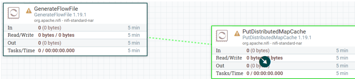
Рисунок 12.13 PutDistributedMapCache
