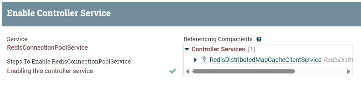
Рисунок 12.7 RedisConnectionPoolService
